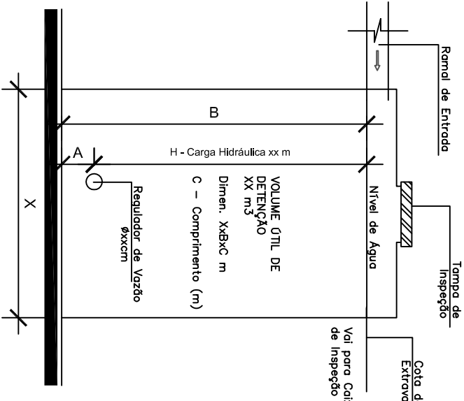
EXQUEMA DO SISTEMA DE DETENÇÃO SEM ESCALA
