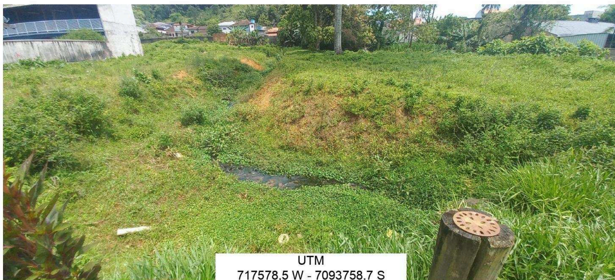
Figura 42: trecho 40 - transição de curso d'água aberto com vegetação isolada para tubulado
