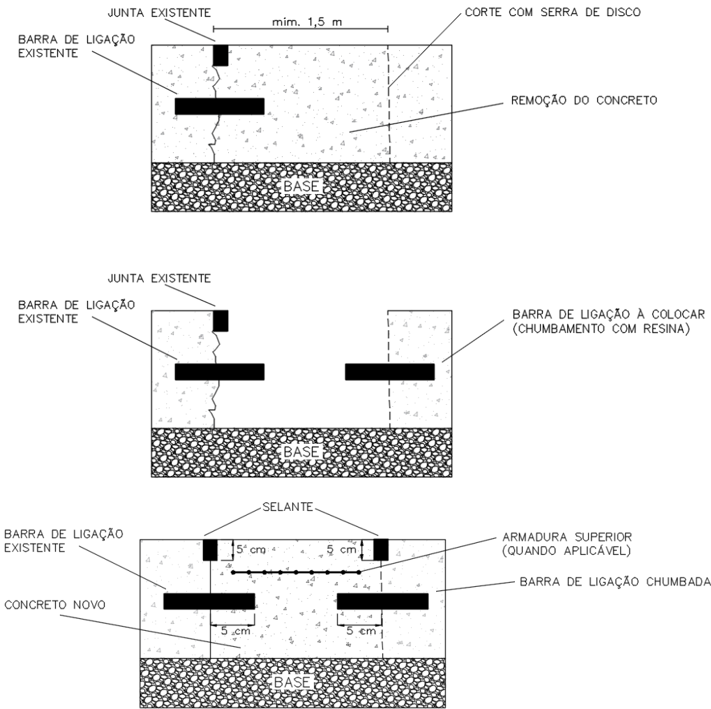
CORTE A-A': SEQUÊNCIA DE EXECUÇÃO
