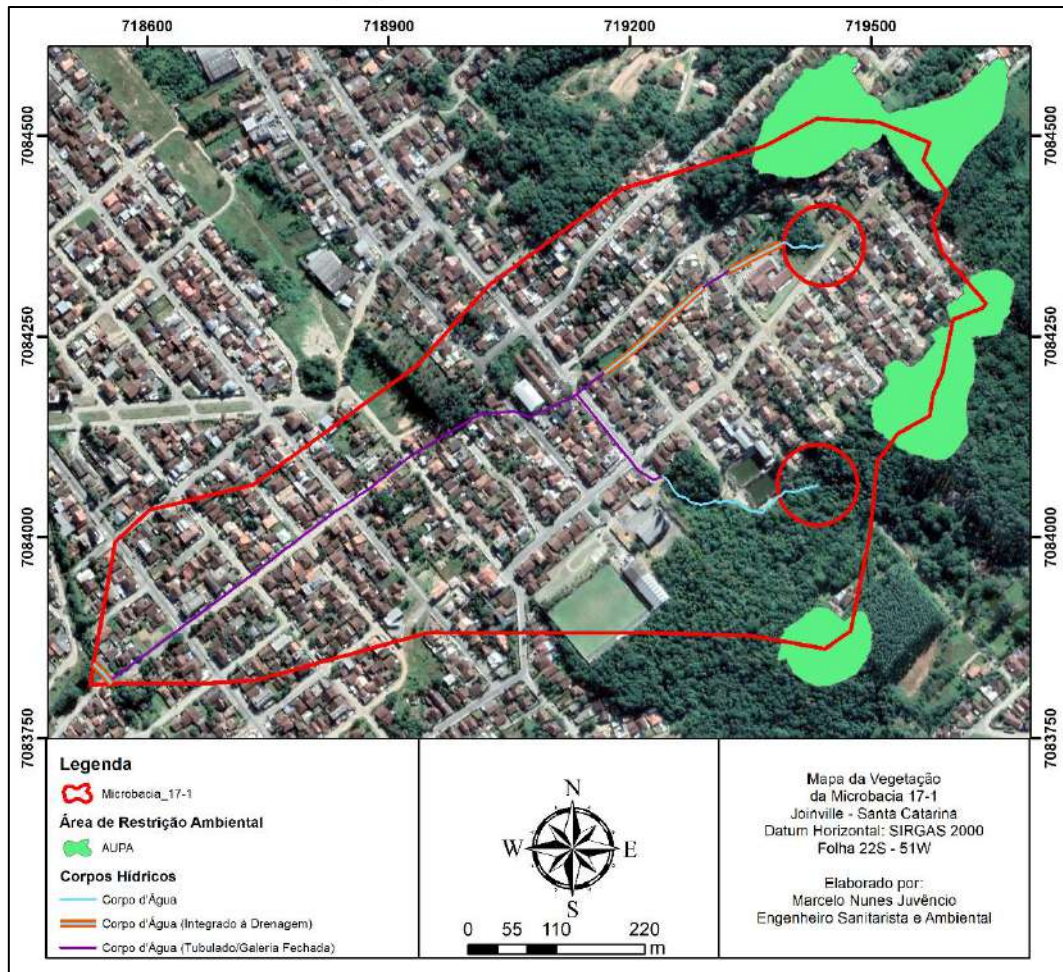
Figura 12 - Área de Restrição Ambiental. Autor: Marcelo Nunes Juvêncio. Data: 21/06/2022.
