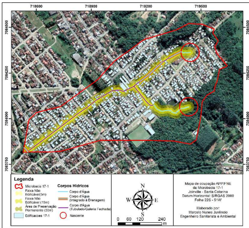
Figura 6 - Ocupação nas faixas de FNE e APP na microbacia 17-1
