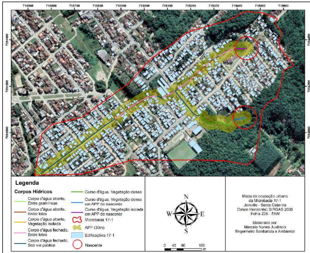
Figura 5 - Mapa de ocupação da Microbacia 17-1 com APP de 30m
