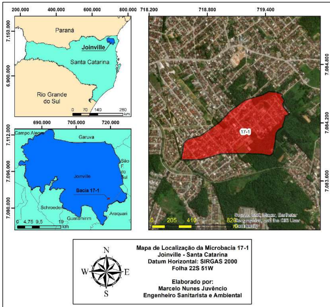
Figura 1 - Localização da Microbacia 17-1
