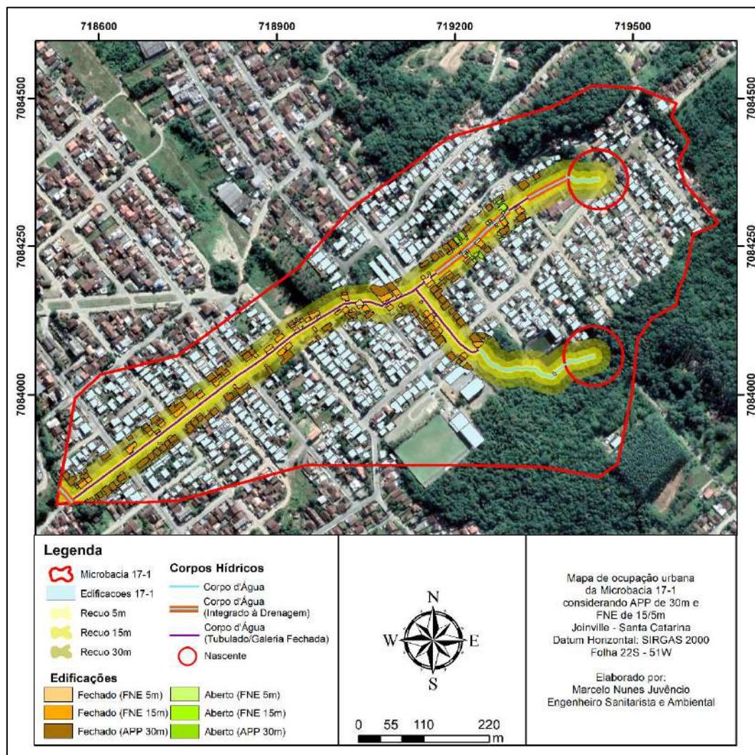
Figura 7 -Áreas edificadas nas faixas marginais dos corpos d'água em canal aberto e fechado. Autor: Marcelo Nunes Juvêncio. Data: 23/05/2022.
