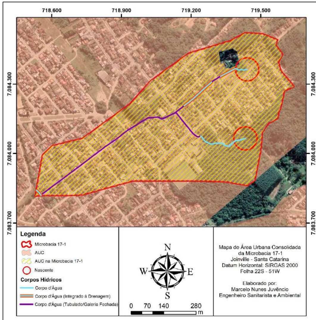
Figura 4 - Área urbana Consolidada na microbacia 17-1.
