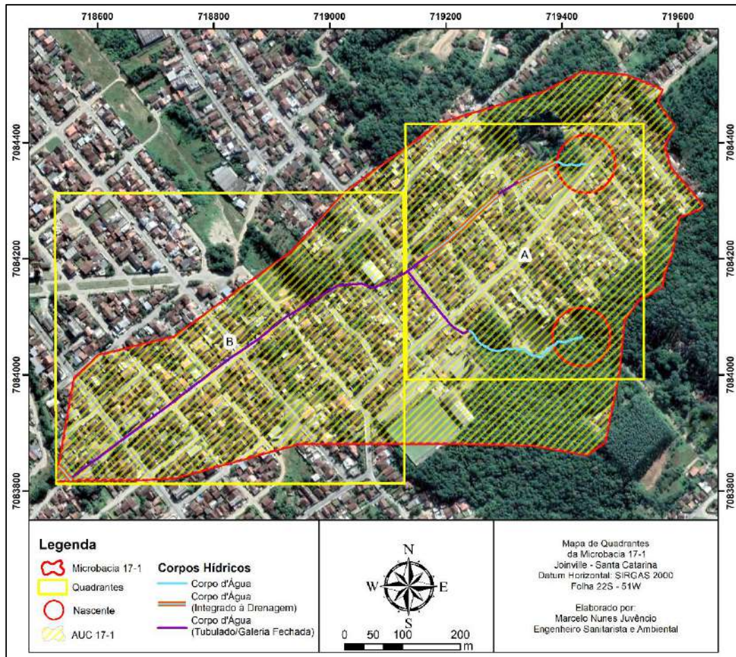
Figura 14 - Quadrantes da Microbacia 17-1. Autor: Marcelo Nunes Juvêncio. Data: 26/05/2022.
