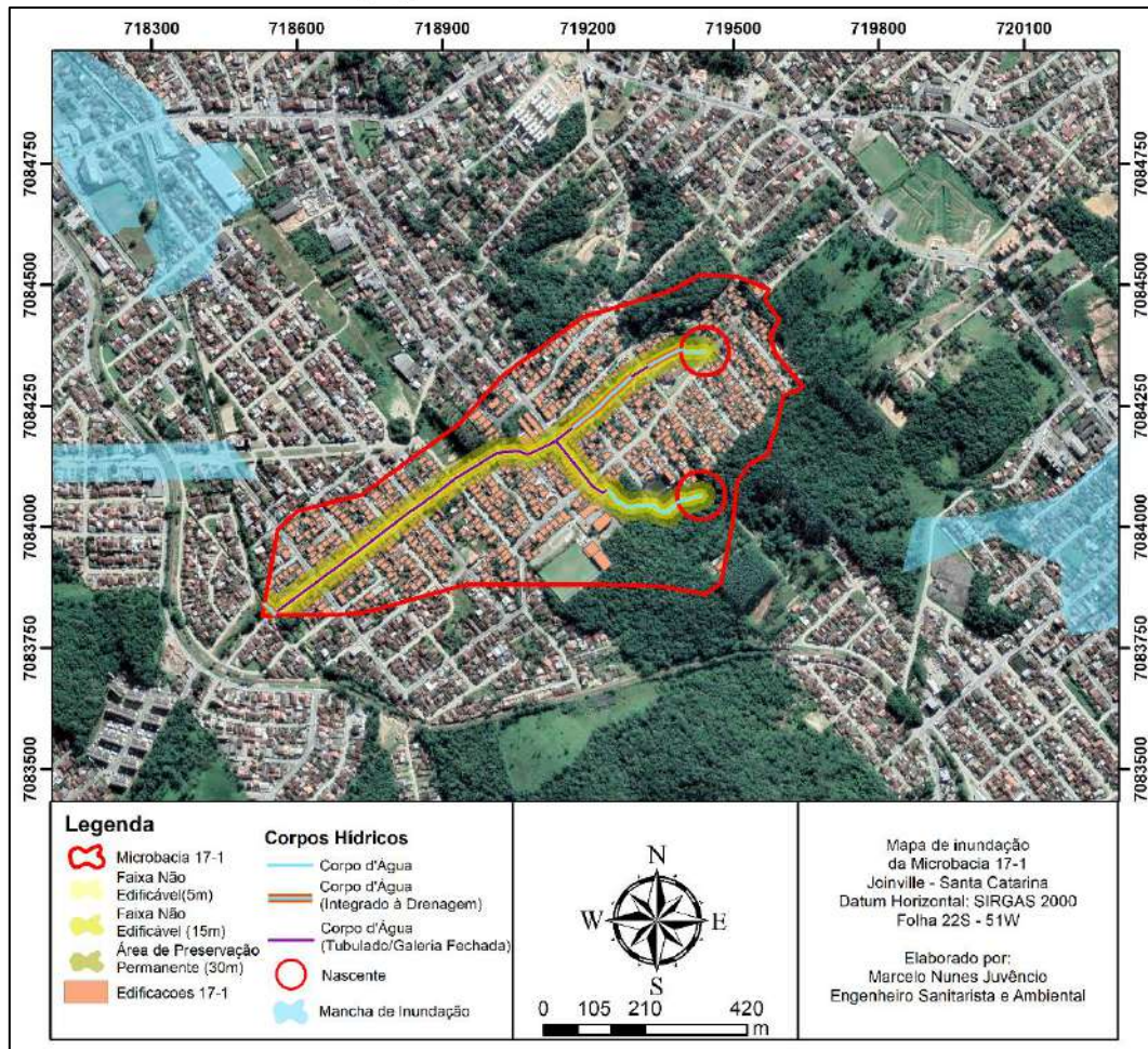
Figura 8 - Mancha de inundação na Microbacia 17-1. Autor: Marcelo Nunes Juvêncio. Data: 24/05/2022.
