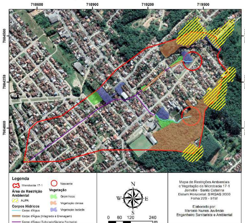
Figura 13 - Áreas vegetadas, restrições ambientais e cursos hídricos na microbacia 17-1. Autor: Marcelo Nunes Juvêncio. Data: 06/10
