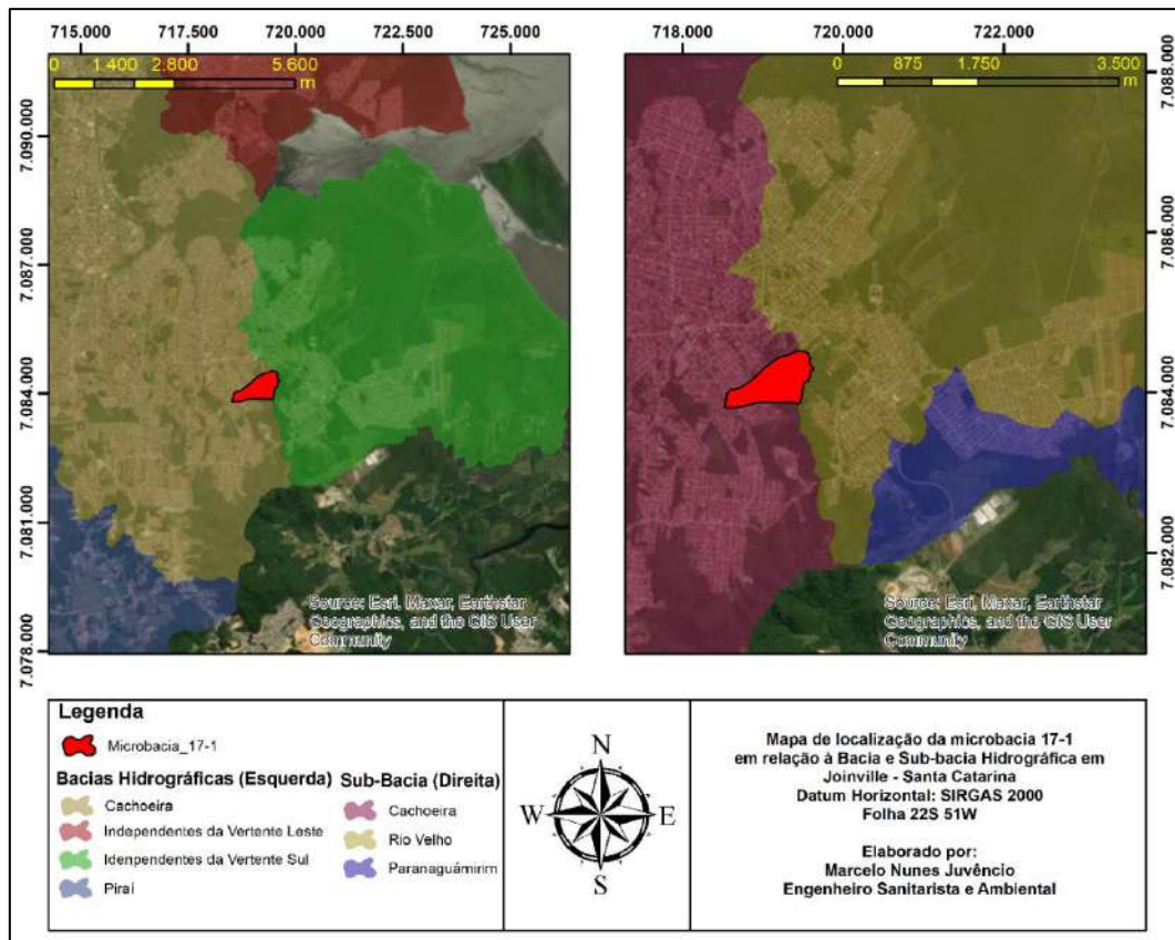
Figura 2 - Bacia e Sub-bacia hidrográfica. Microbacia 17-1
