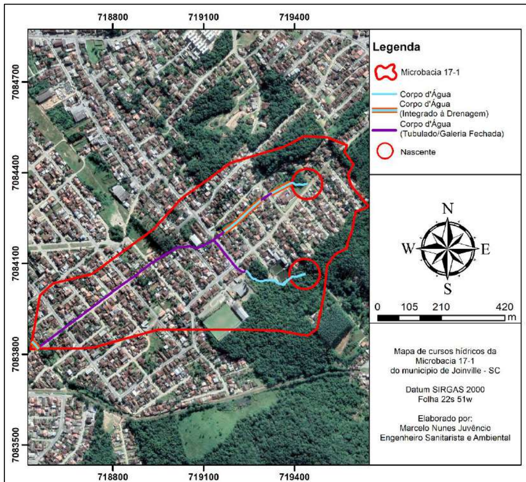
Figura 3 - Corpos hídricos na Microbacia 17-1.
