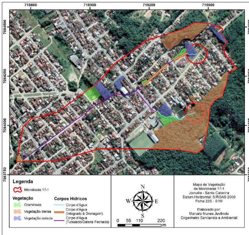
Figura 11 - Vegetação na Microbacia 17-1. Autor: Marcelo Nunes Juvêncio. Data: 06/10/2022.
