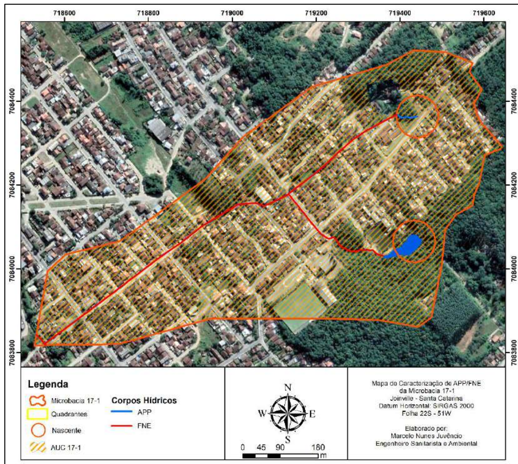
Figura 40 - Caracterização dos corpos hídricos na Microbacia 17-1.
